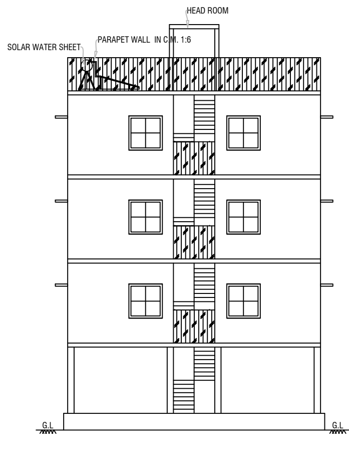
ELEVATION
