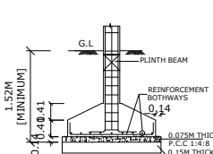
TYP. DET. COLUMN FOOTING
