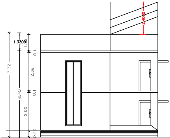
ELEVATION
