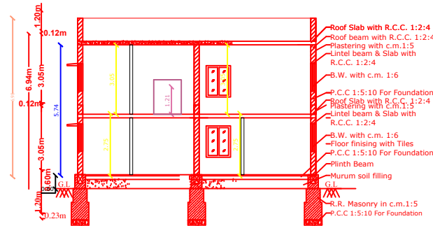
SECTION 'AB'
