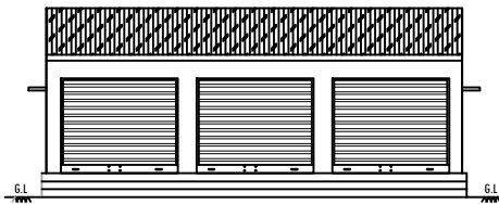
ELEVATION
