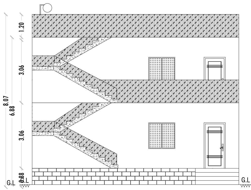
ELEVATION
