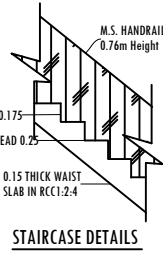
STAIRCASE DETAILS SCALE: 1:20
