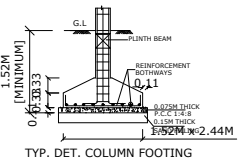
TYP. DET. COLUMN FOOTING
