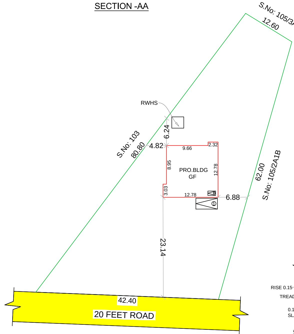
SITE PLAN SCALE: 1:400
