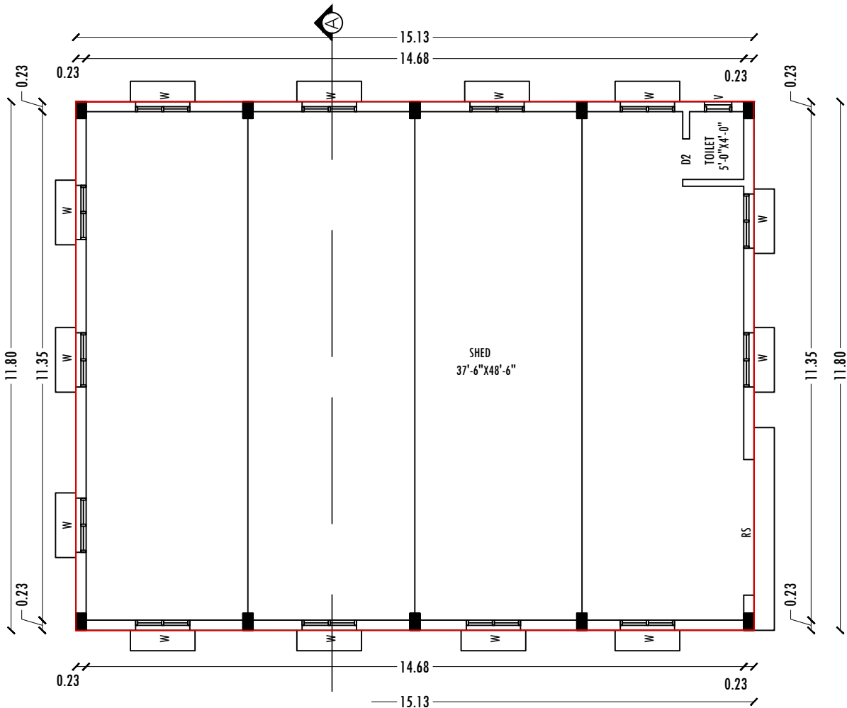
D PLAN
