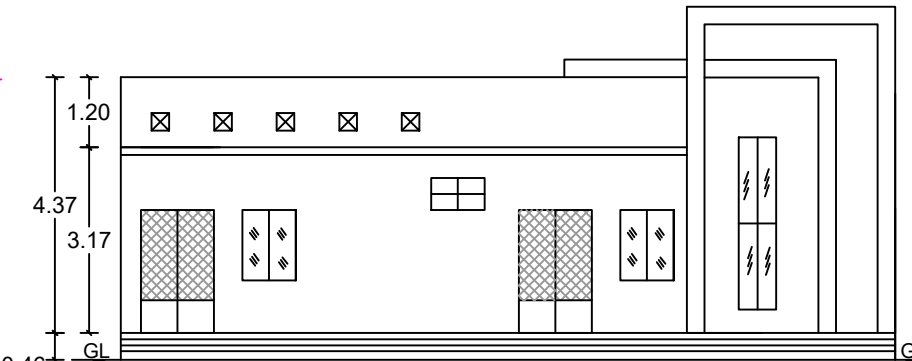
ELEVATION
