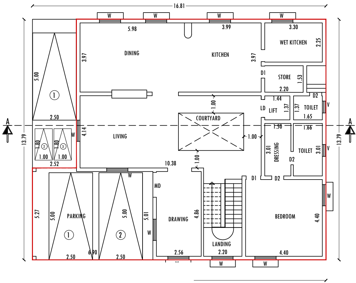
DR PLAN
