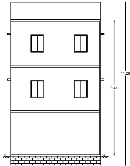
ELEVATION
