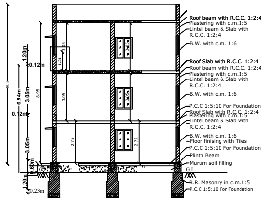
SECTION 'AB'
