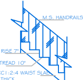
STAIRCASE DETAILS SCALE: 1:20
