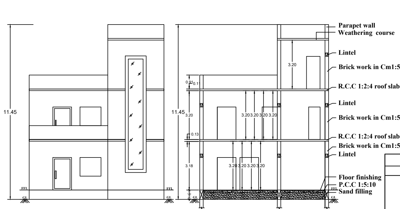
ELEVATION
