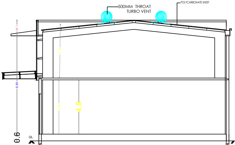
SECTION A-B
