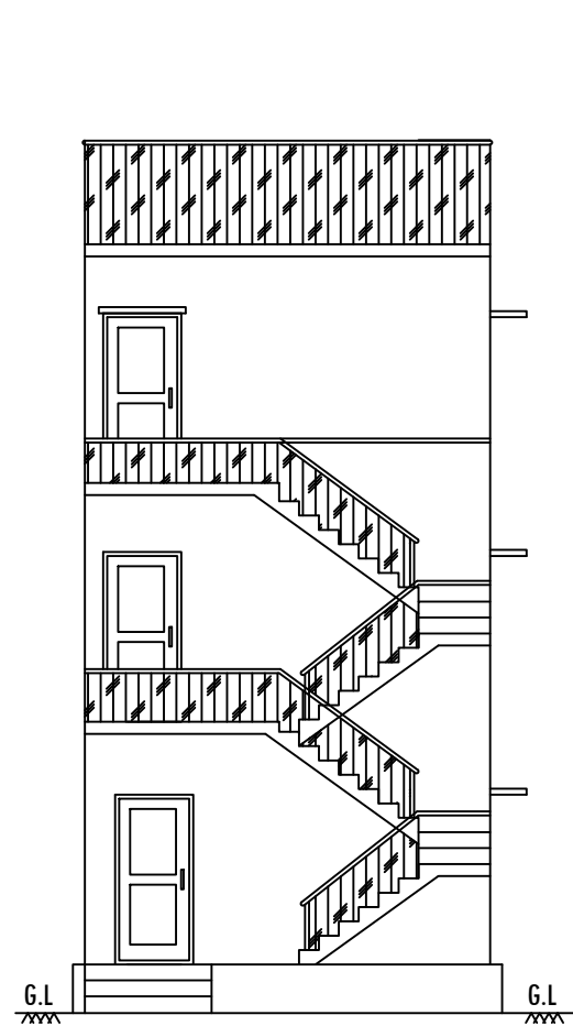
ELEVATION
