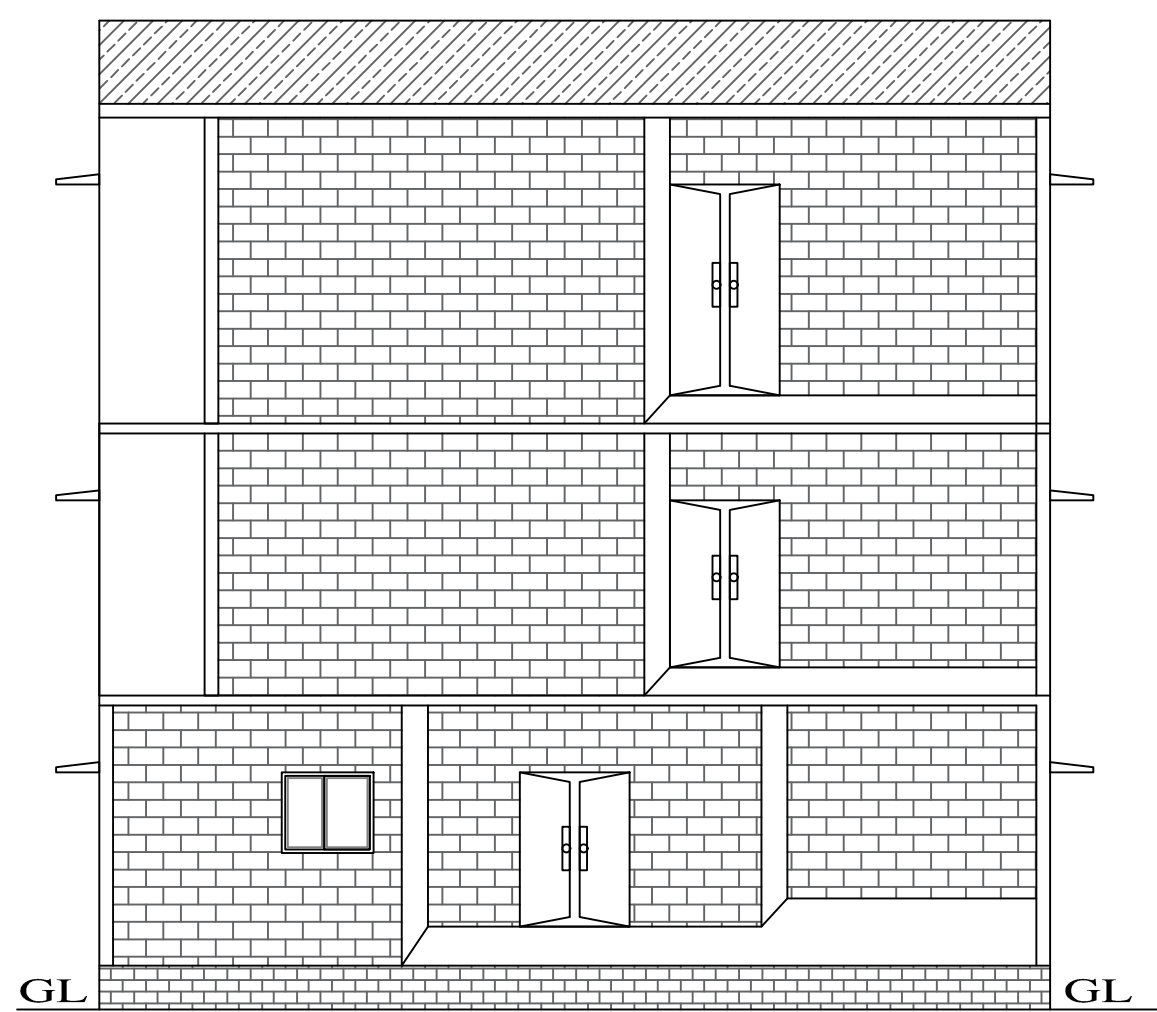
ELEVATION
