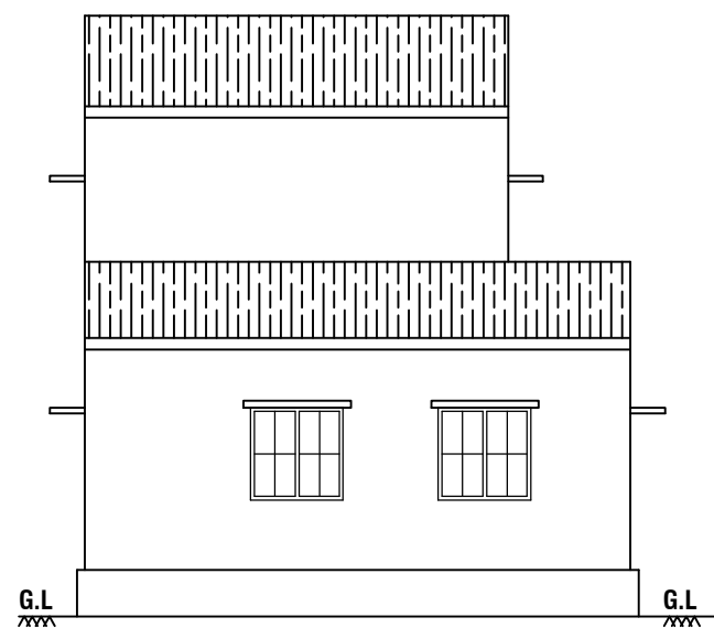
ELEVATION
