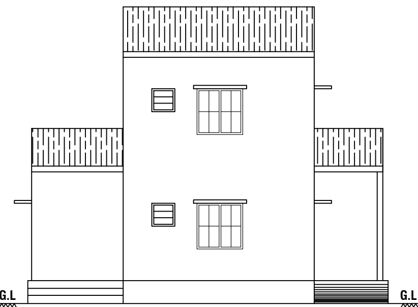
ELEVATION
