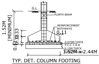
TYP. DET. COLUMN FOOTING
