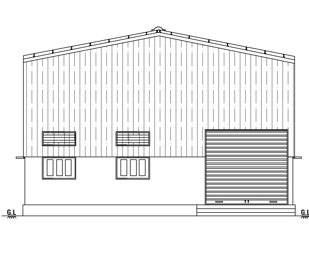
ELEVATION
