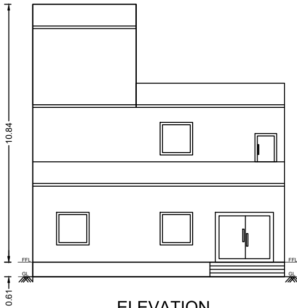
ELEVATION
