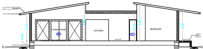
SECTION AA' (IN FT & IN) SCALE - N.T.S.
