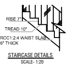
STAIRCASE DETAILS SCALE: 1:20
