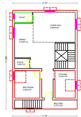
PRO.FIRST FLOOR PLAN SCALE: 1:100
