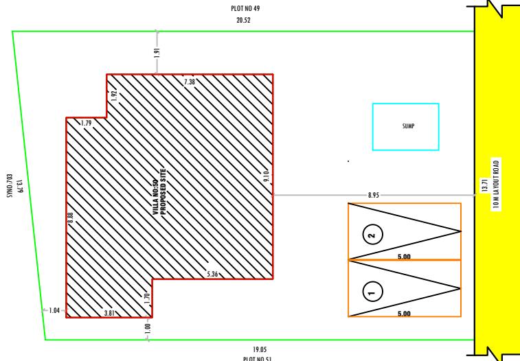
SITE PLAN - 1:100
