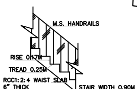
STAIRCASE DETAILS SCALE: 1:20
