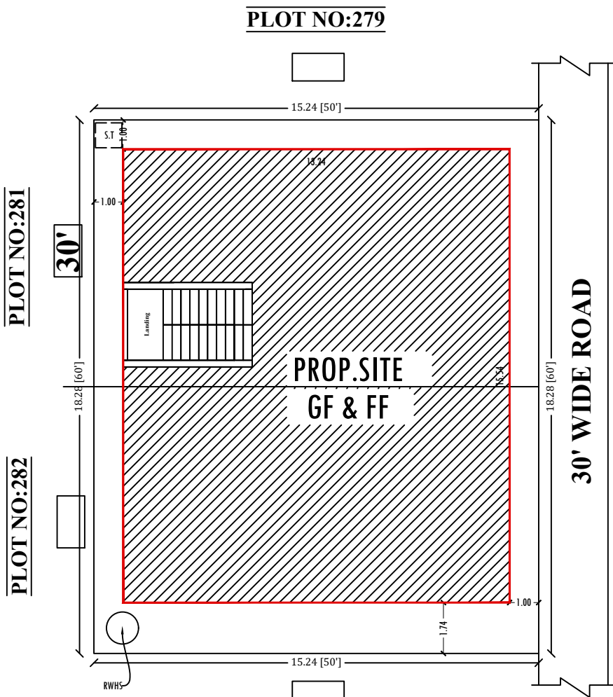
SITE PLAN(SCALE: 1:100)
