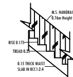
STAIRCASE DETAILS SCALE: 1:20
