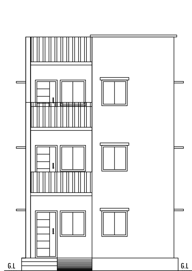
ELEVATION
