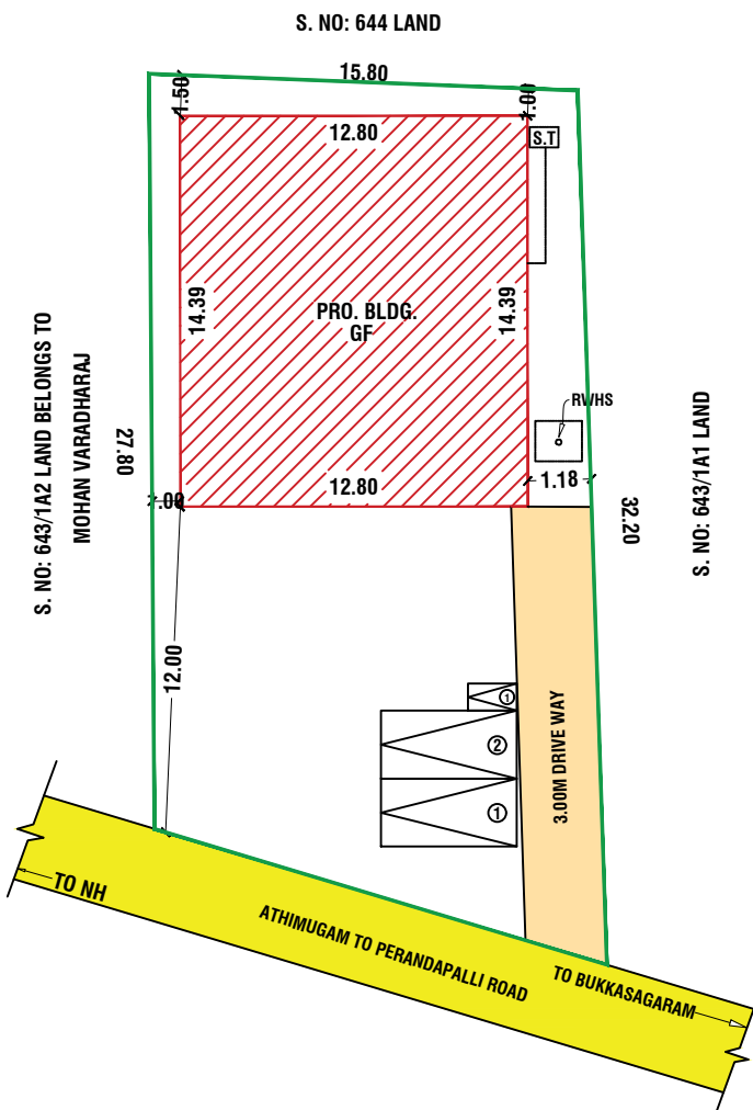
SITE PLAN SCALE: 200
