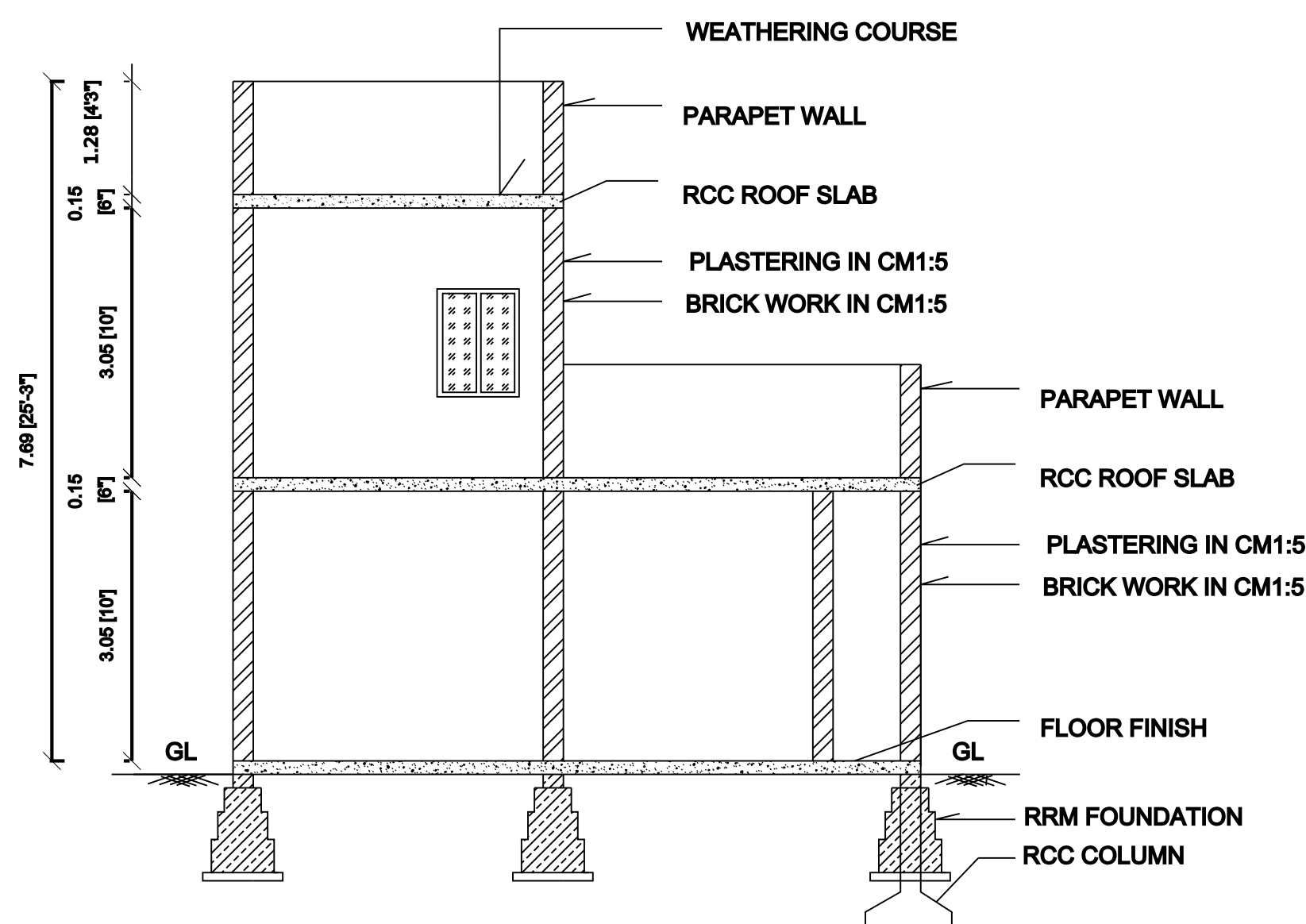
SECTION - AA' - BB'
