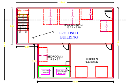
PRO. FIRST FLOOR PLAN SCALE: 1:100
