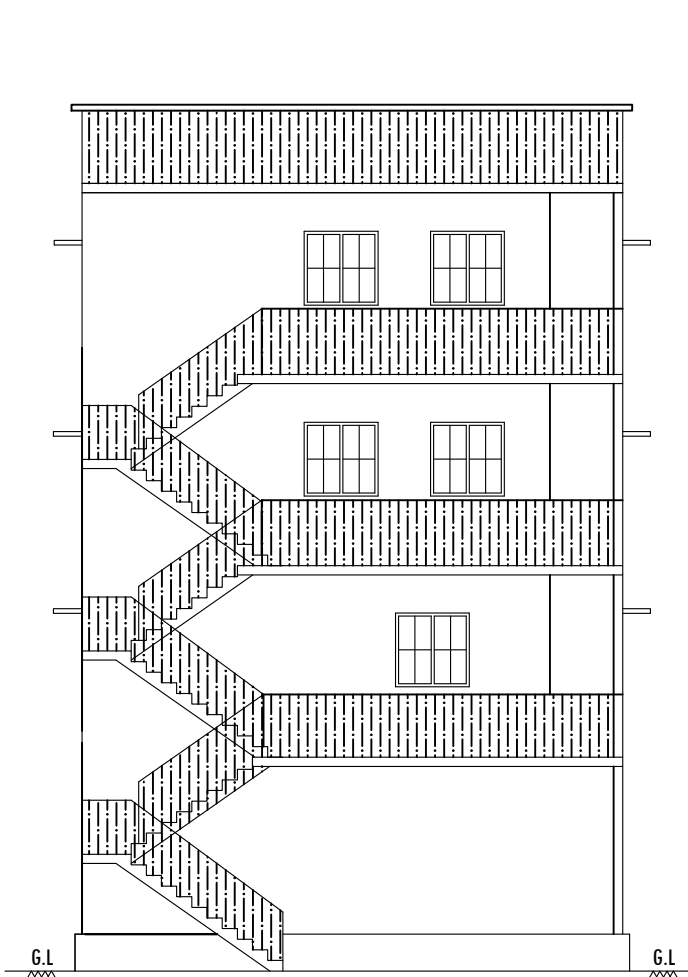
ELEVATION
