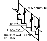
STAIRCASE DETAILS SCALE: 1:20
