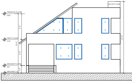
ELEVATION 1
