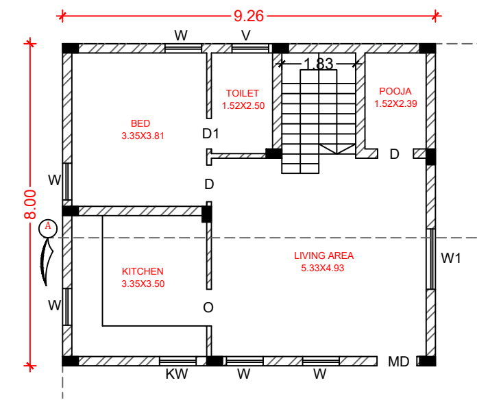
UND FLOOR (BLOCK -1)
