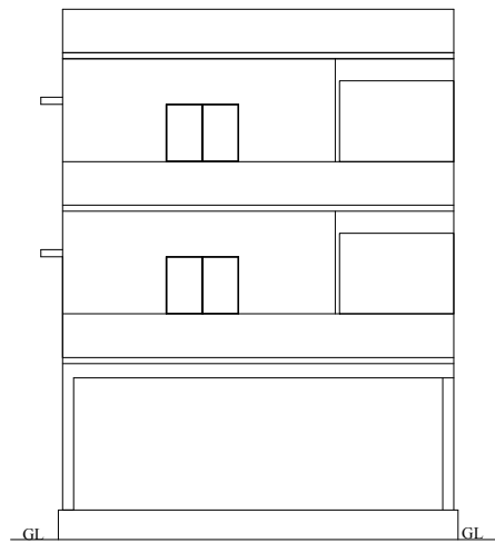
ELEVATION
