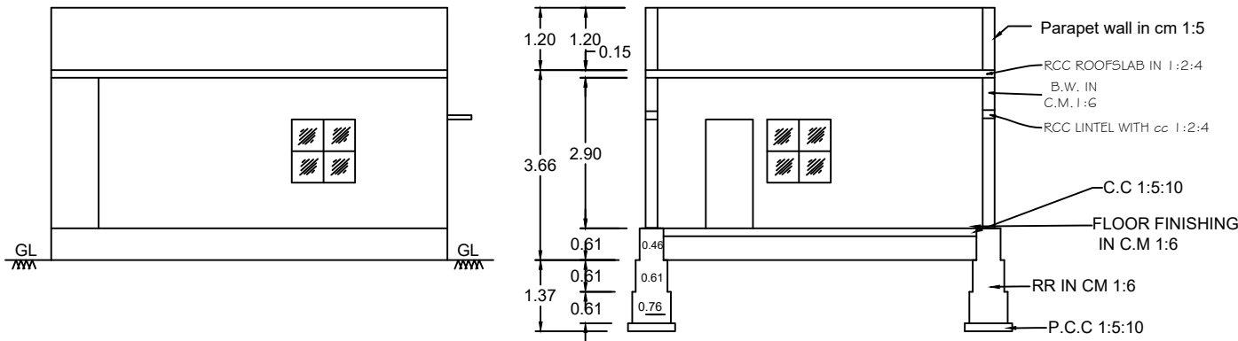
ELEVATION
