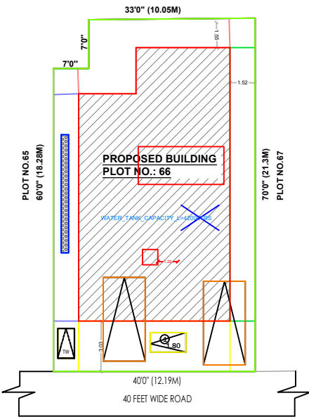
SITE PLAN.
