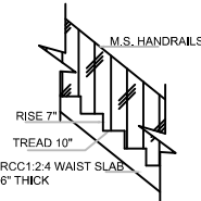
STAIRCASE DETAILS SCALE: 1:20
