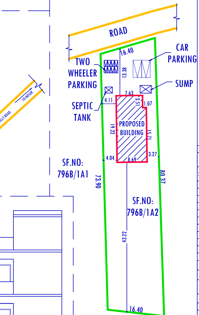
SITE PLAN (SCALE - 1:400)
