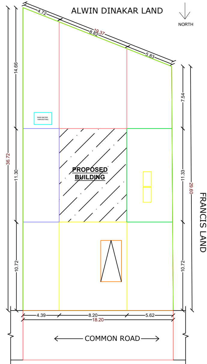
SITE PLAN 1 : 100
