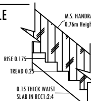
STAIRCASE DETAILS SCALE: 1:20
