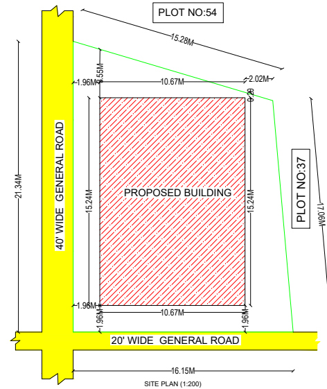
SITE PLAN (1:200)
