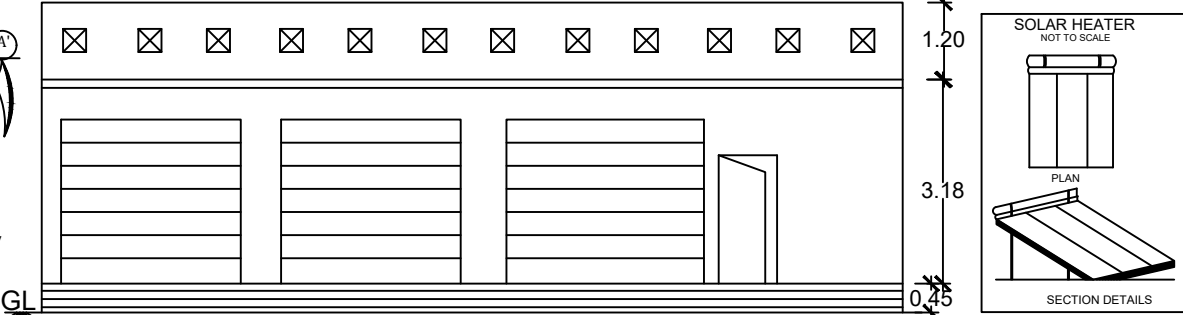
ELEVATION
