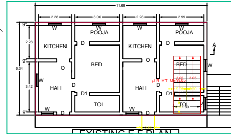
EXISTING F.F PLAN
