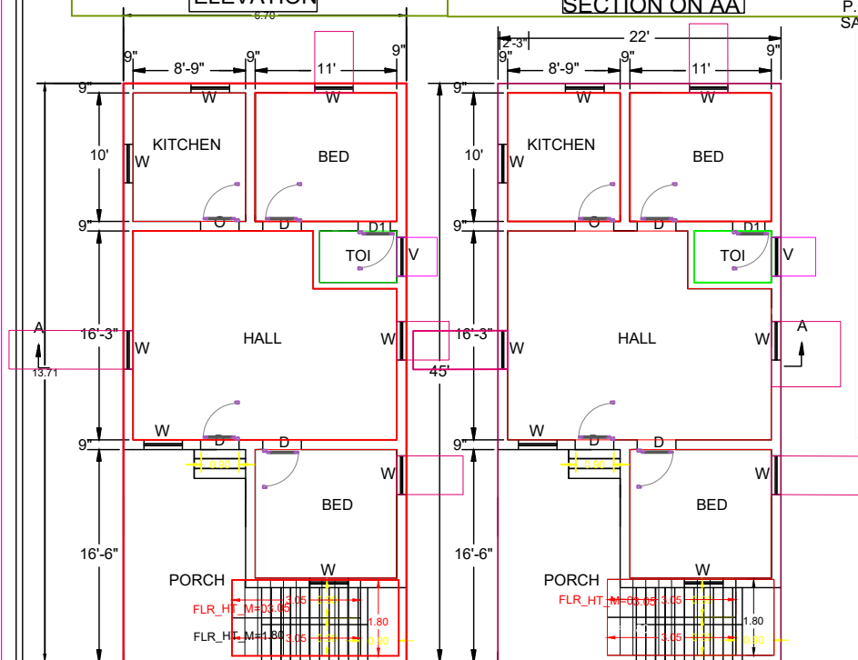
G.F PLAN
