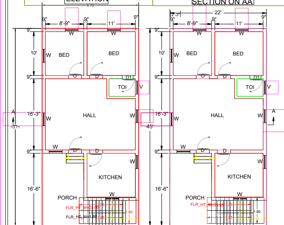
G.F PLAN
